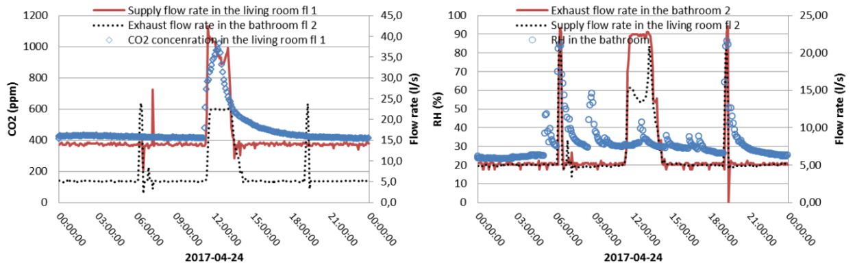
Figur 2. Uppmätta halter av CO 2 , RH samt till- och frånluftsflöden. (Hämtat från RISE rapport)
