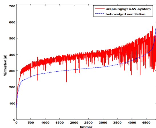
Figur 4. Varaktighetsdiagram för det behovsstyrda ventilationssystemet tillsammans med CAV-systemet. (Hämtat från RISE rapport)
