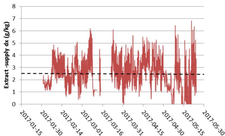
Figur 3. Uppmätt fukttillskott januari-maj 2017 i Forskningsvillan. (Hämtat från RISE rapport)
